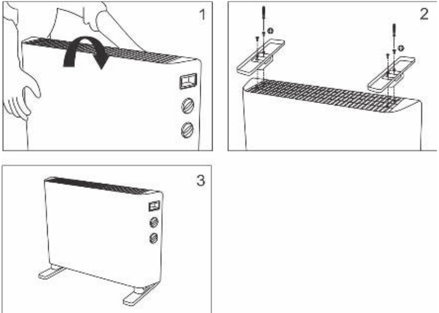
Рис. 1. Напольная установка
